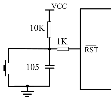
图 9-2 建议 \overline{\text{RST}} 复位电路
