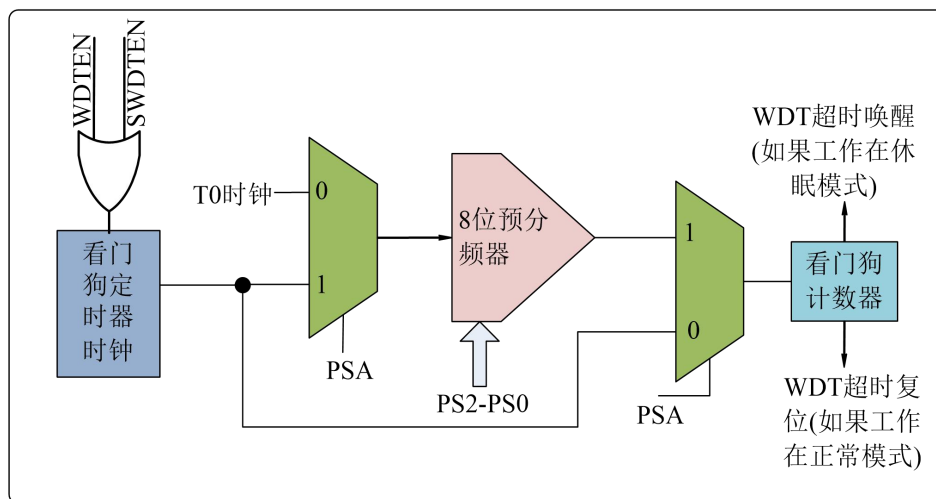
图 11-1 看门狗定时器框图
