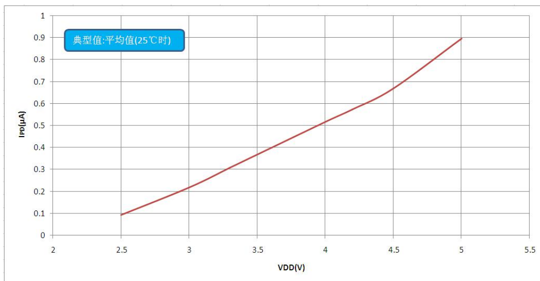
图 13-2：不同 VDD 时典型 I PD — VDD 关系曲线图
